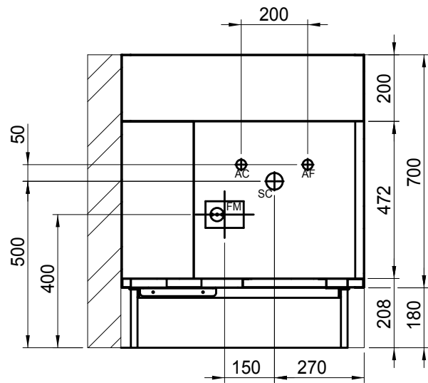
SEZIONE B-B
