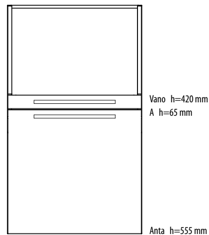
Modulo per termosigilatrice Lowered module for autoclave Module surbaissé pour autoclave Gesenktes Modul für Autoklav Módulo bajo para autoclave
