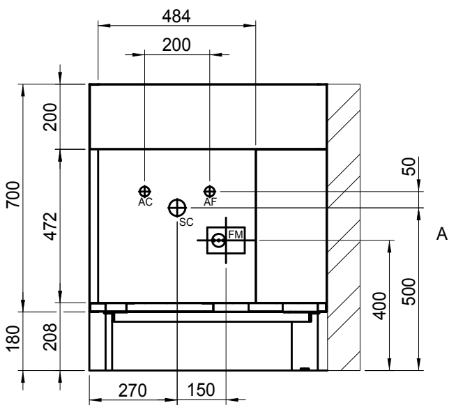
SEZIONE A-A
