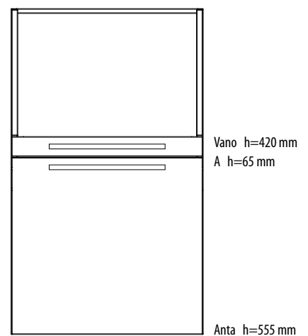
Modulo per termosigilatrice
